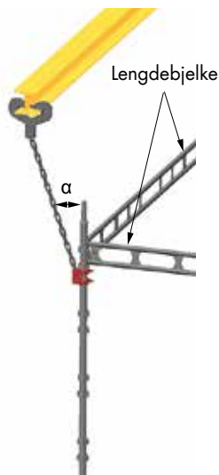
Lasttilfelle 1: Tillatte laster som funksjon av vinkelavvik
