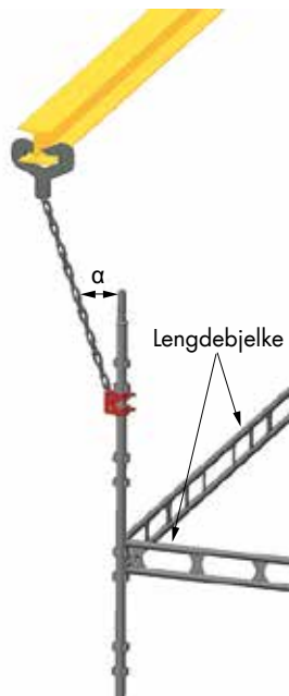
Lasttilfelle 3: Bøyemoment som funksjon av vinkelavvik
