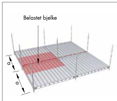
Utbreidd stillas
